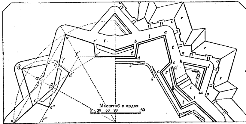
ЧЕРТЕЖ 1
